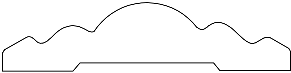
B-801 1 1/16" X 3"
